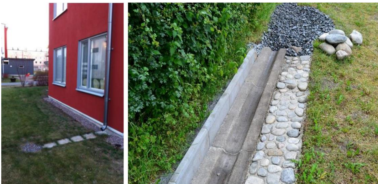
Figur 6-8. Utkastare med rännal som leder vattnet till små stenistor i gräsmattan, exempel från Märsta i Sigtuna kommun, (T,h,). Dagvattnet når stenistan via en dagvattenränna, för hus utan källare rekommenderas att perkolationsmagasin anläggs minst två meter från huset, för hus med källare rekommenderas minst fem meter. Foto: poppelhus,se.
