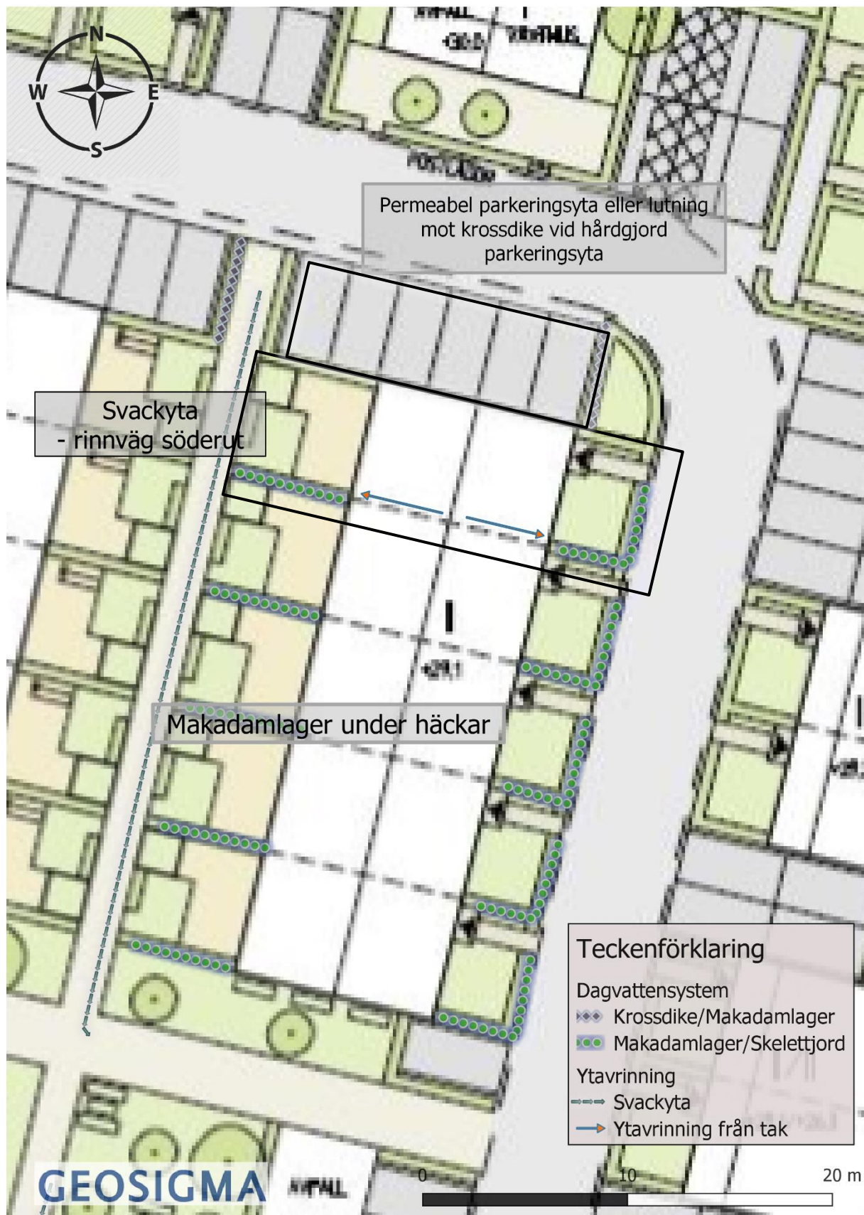
Figur 6-3. Schematisk skiss över föreslaget dagvattensystem.
