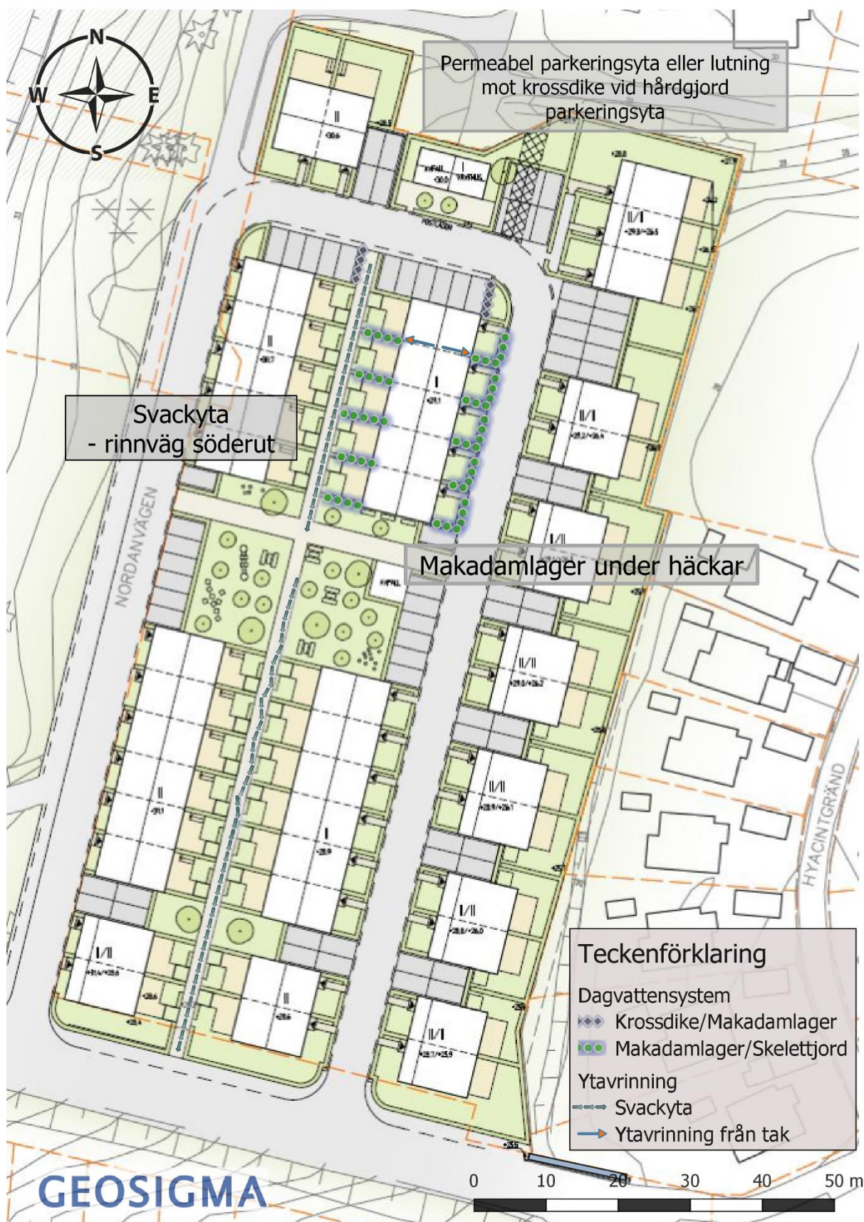
Figur 6-1. Schematisk skiss över föreslaget dagvattensystem med makadamlager/skelettjord under häckarna längs tomterna och parkeringarna. Kompletterande krossdiken eller permeabel yta föreslås vid parkeringarna.
