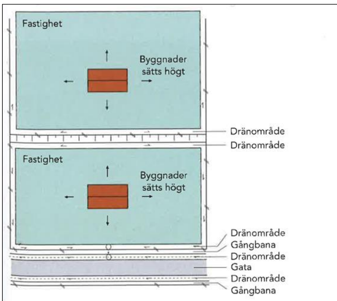
Figur 8-3. Höjdsättningsförslag enligt Svensk vattens publikation P105.
