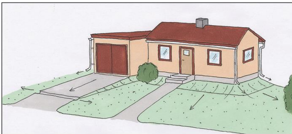
Figur 6-9. Rekommenderad höjsättning för ett bostadshus.
